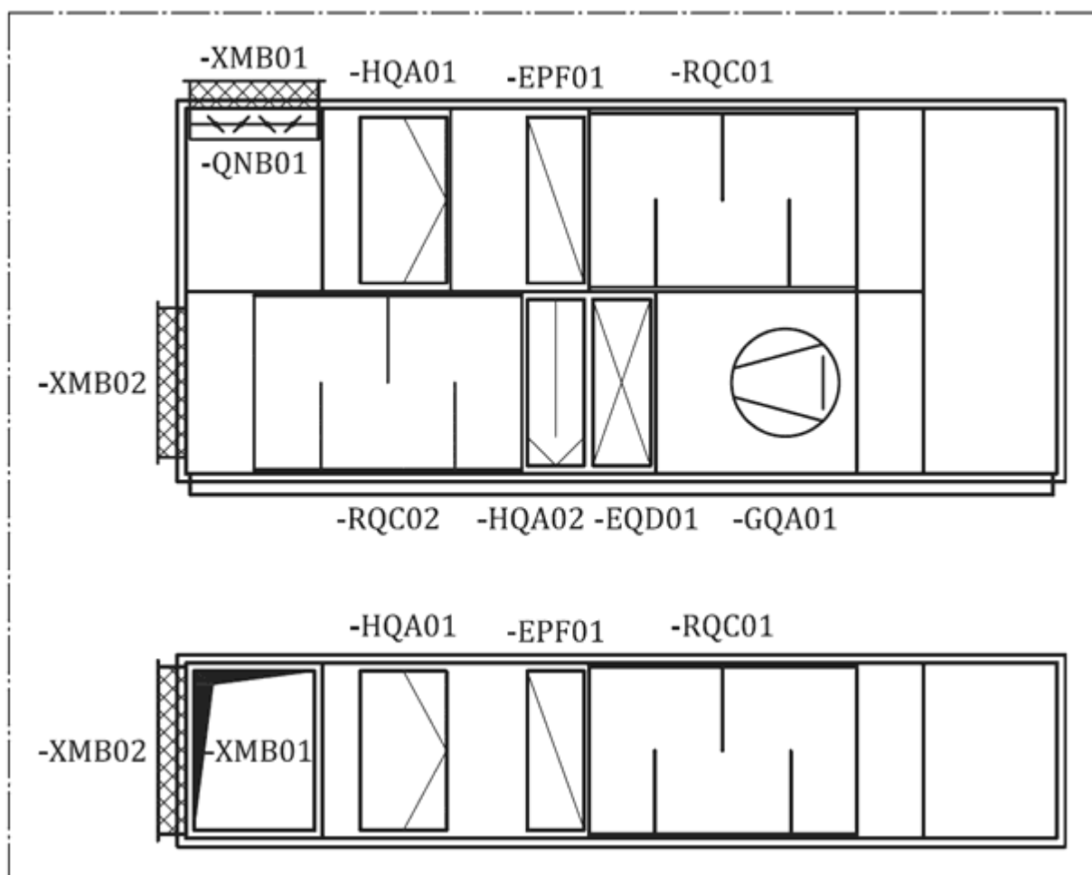
Рисунок В.12 - Схема вентиляционной установки
