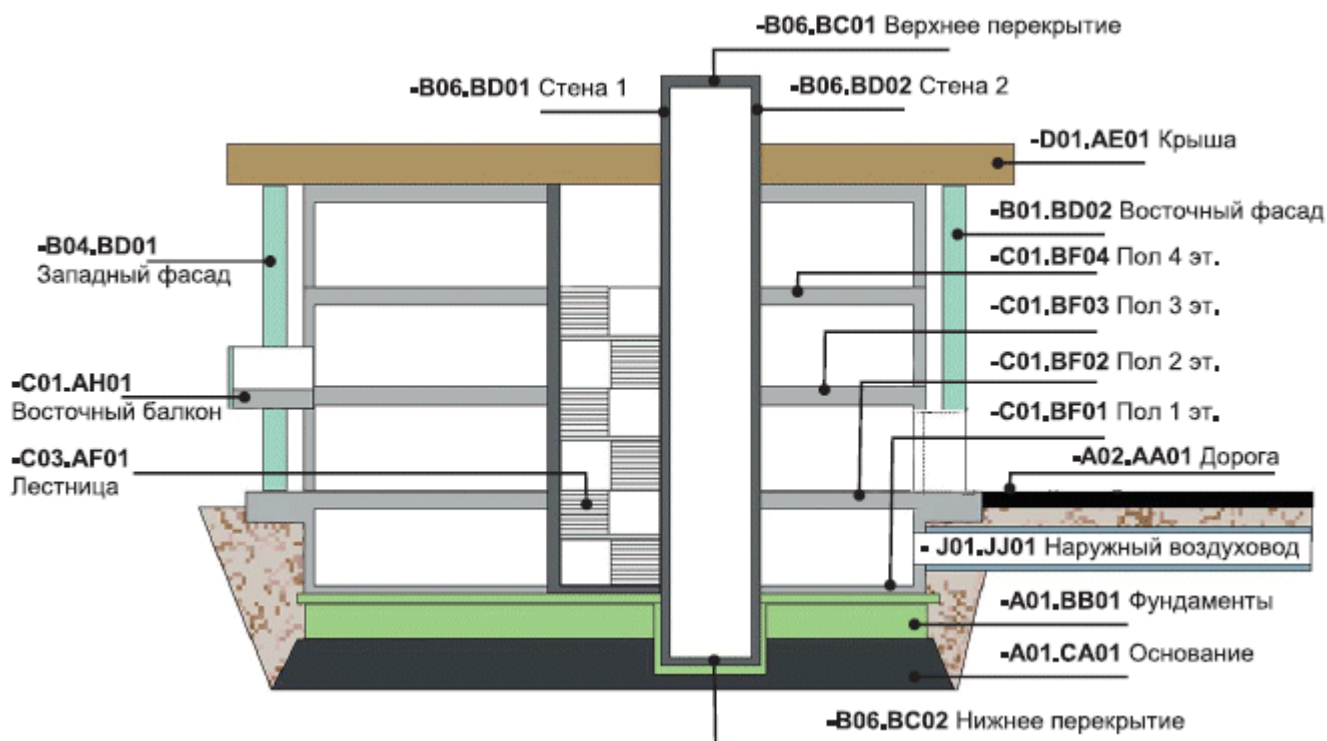
Рисунок В.9 - Обозначение элементов здания на чертеже разреза В.2.2 Виды компонентов и подкомпонентов строительных объектов
