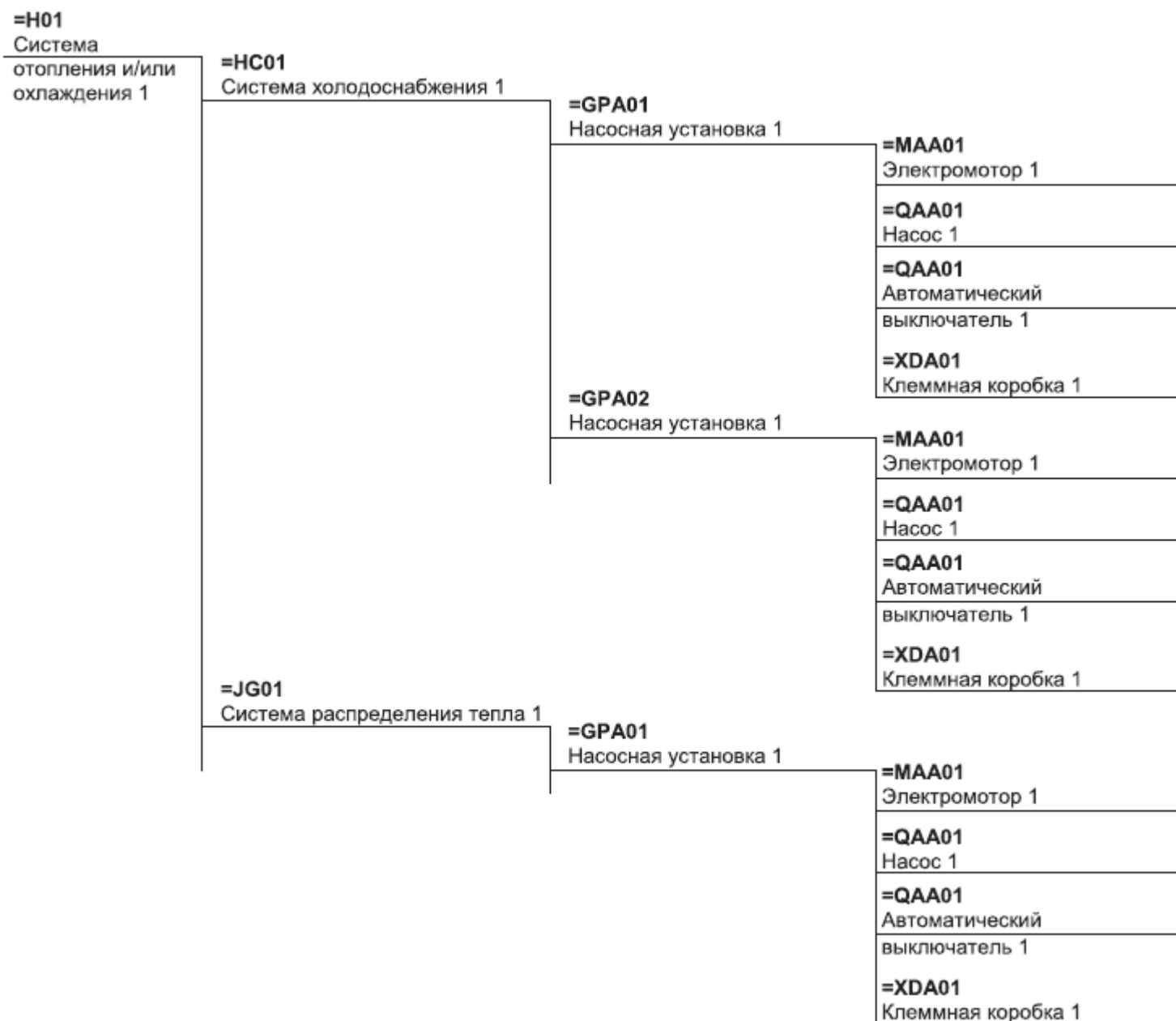
Рисунок В.24 - Древовидная функционально-ориентированная структура представления системы электроснабжения насосных установок
