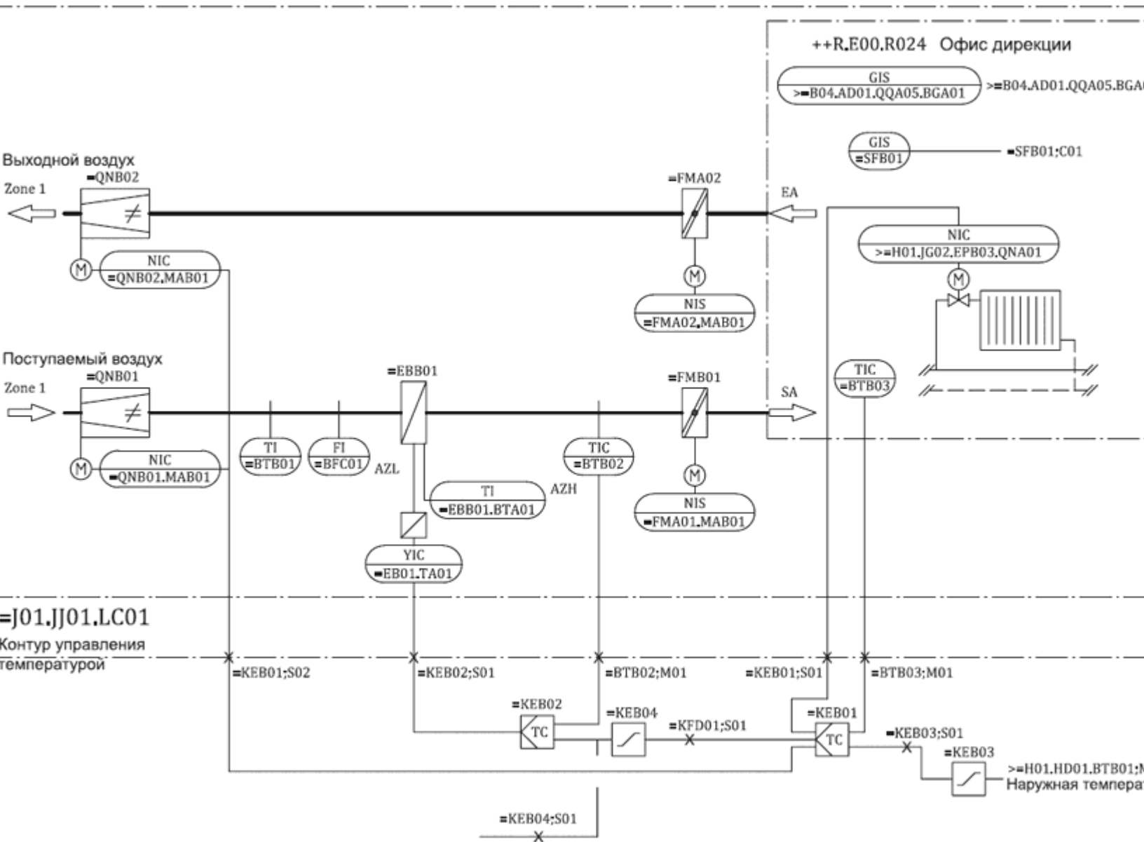
Рисунок В.14 - Схема распределенной системы управления инженерными системами помещения
