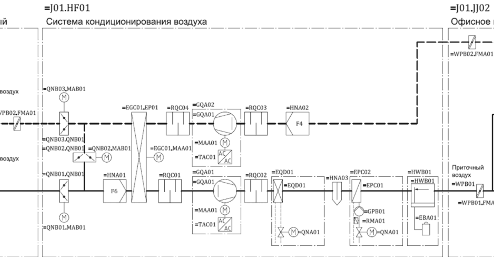
Рисунок В.11 - Принципиальная схема системы ОВиК
