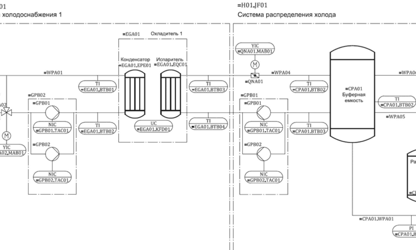
Рисунок В.16 - Принципиальная схема системы холодоснабжения
