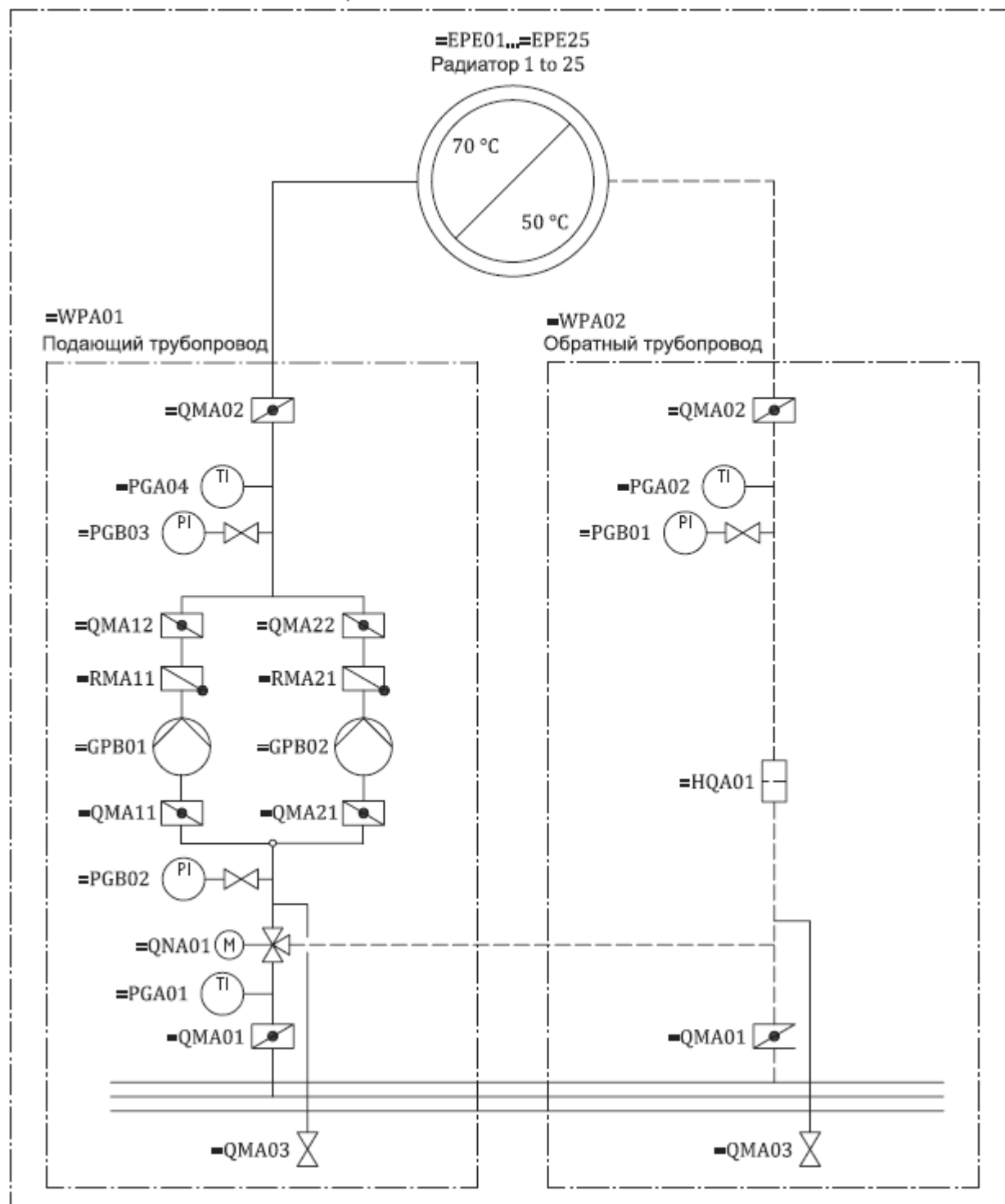
Рисунок В.17 - Принципиальная схема системы отопления
