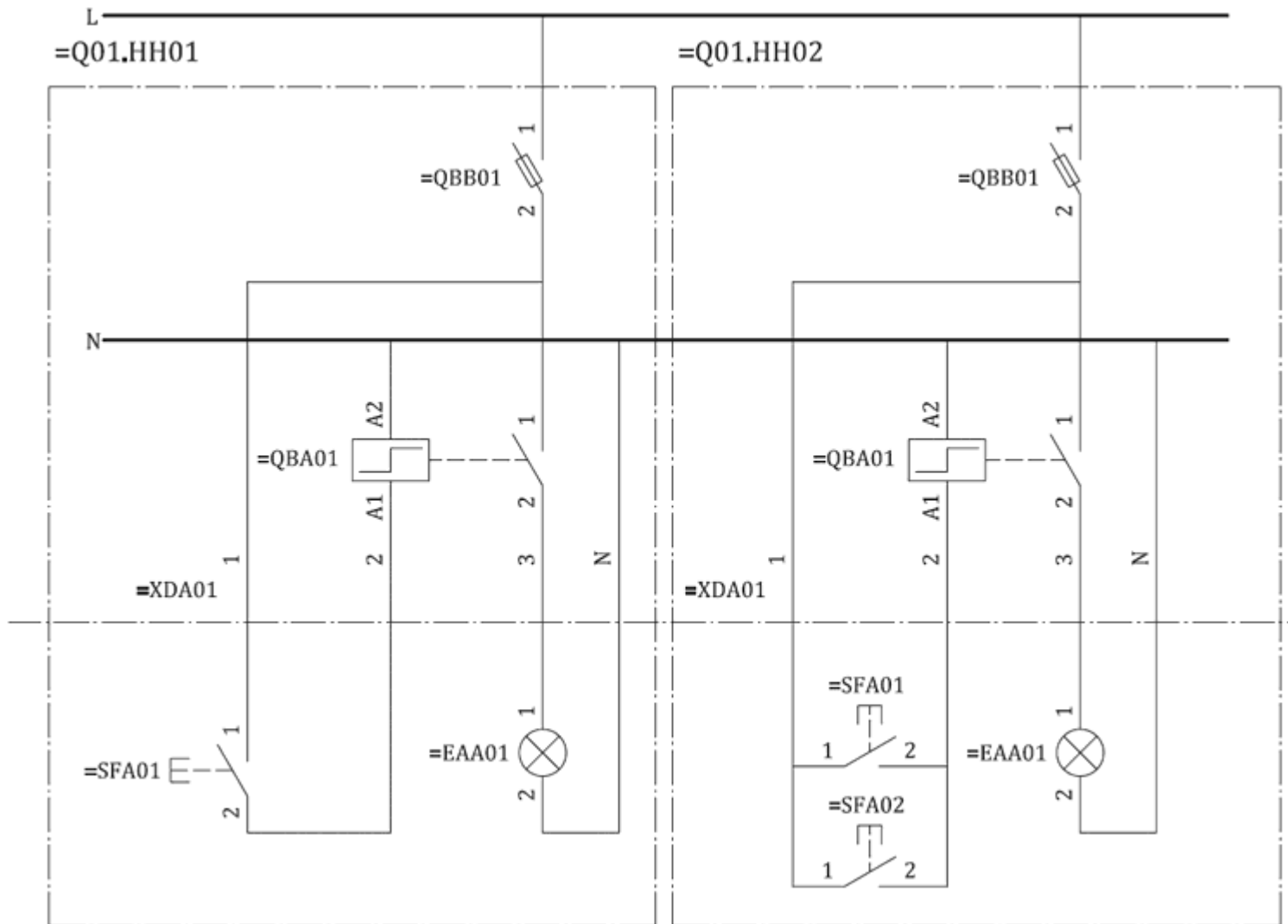
Рисунок В.21 - Схематичное отображение объектов системы освещения
