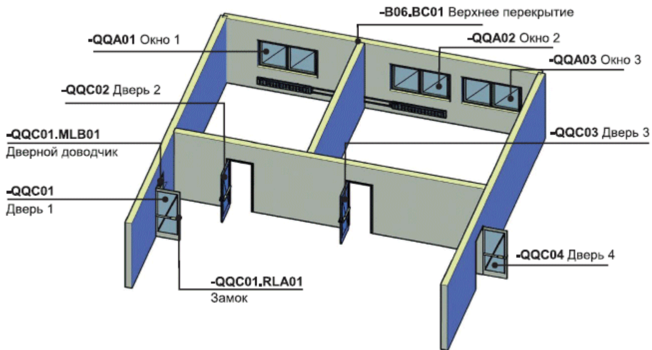
Рисунок В.10 - Обозначение компонентов и подкомпонентов здания
